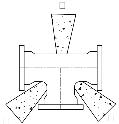
TEE
